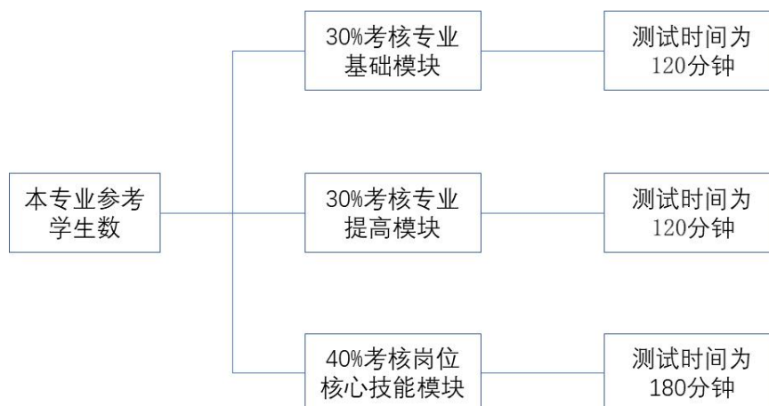
图1 E-R图
