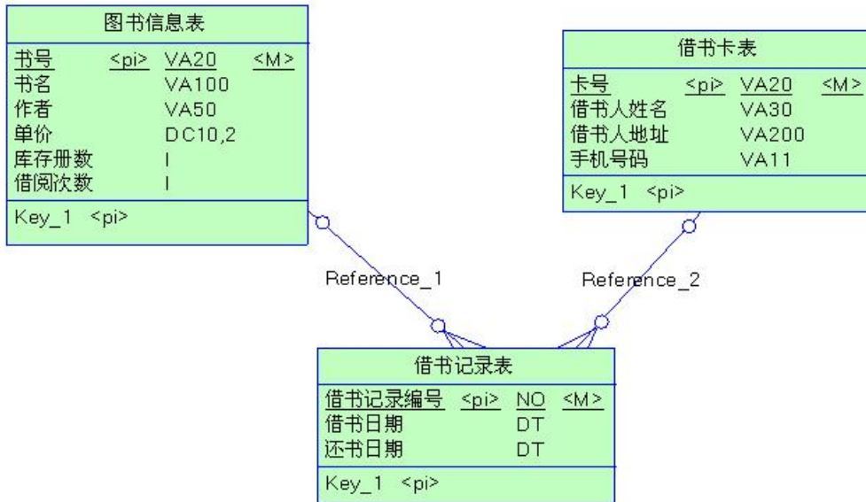
图 2.15.2 逻辑数据模型
