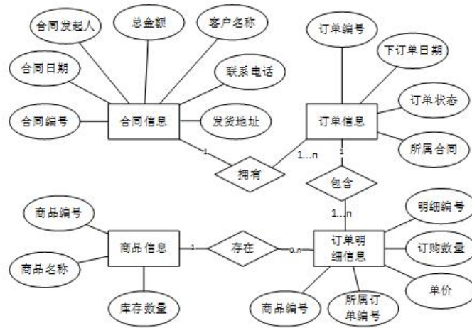
图 2.13.1 E-R 图
