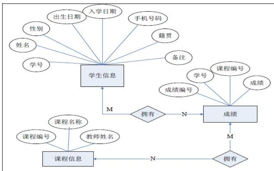
图 2.6.1 E-R 图
