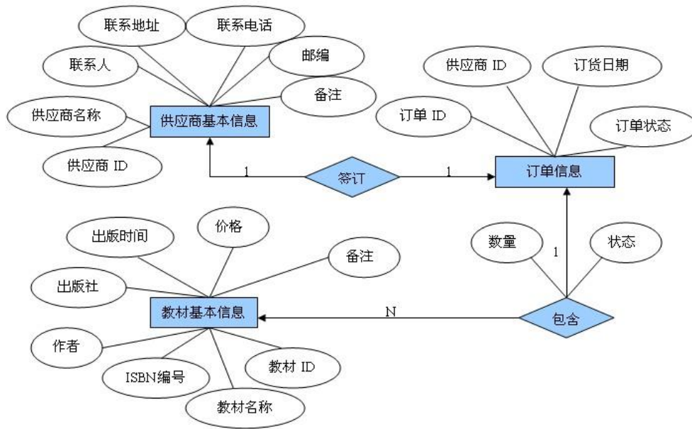
图 2.10.1 E-R 图
