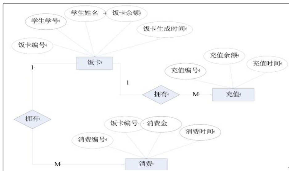
图 2.3.1 E-R 图
