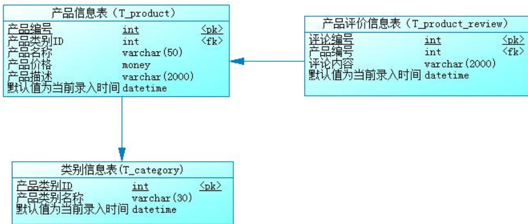
图 2.1.3 物理数据模型图
