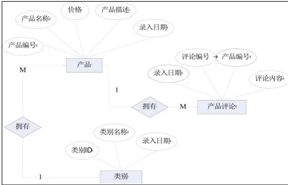
图 2.2.1E-R 图
