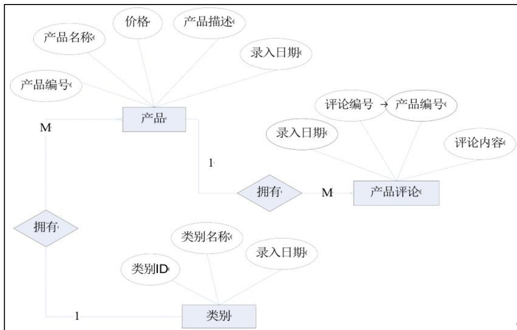
图 2.1.1 E-R 图
