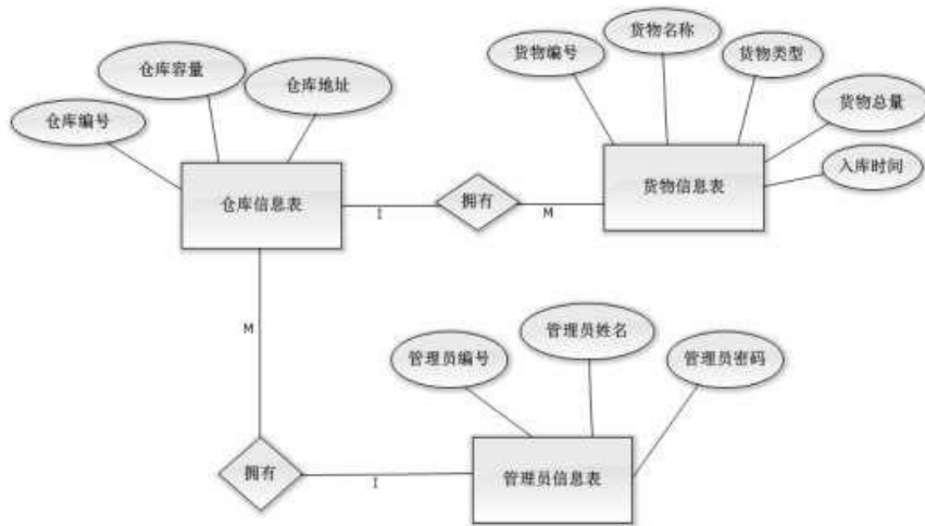
图 2.14.1 E-R 图
