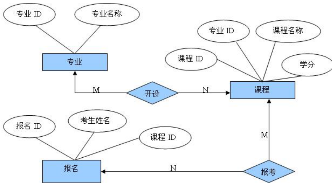
图 2.8.1 E-R 图
