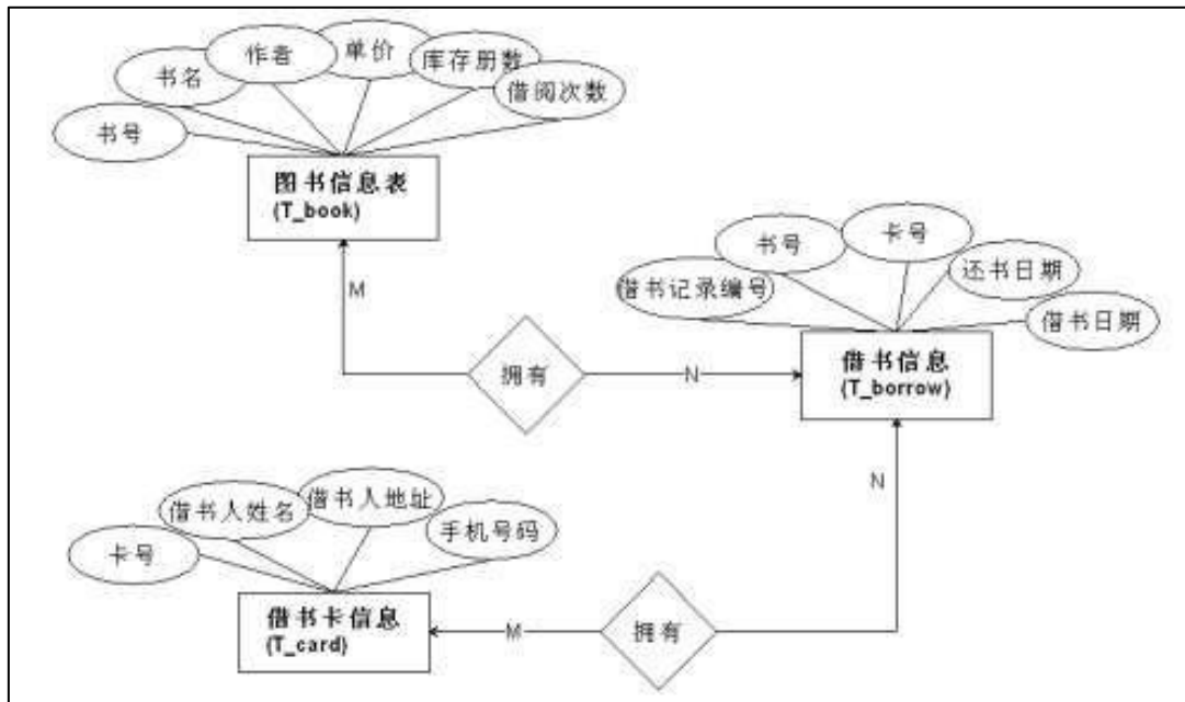
图 2.7.1E-R 图
