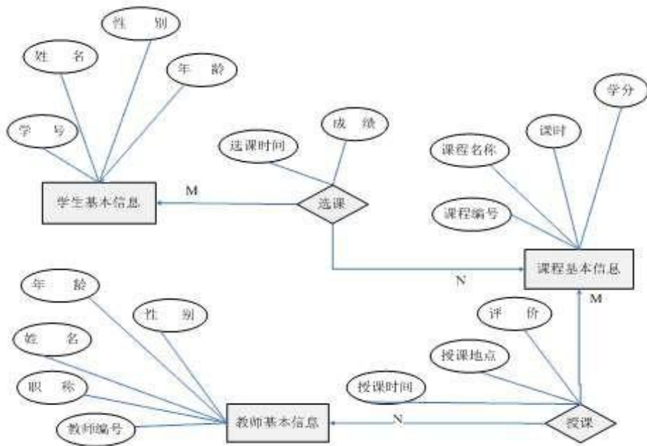
图 2.11.1 E-R 图
