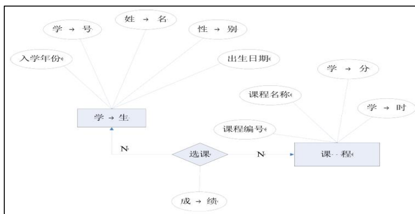
图 2.5.1 E-R 图
