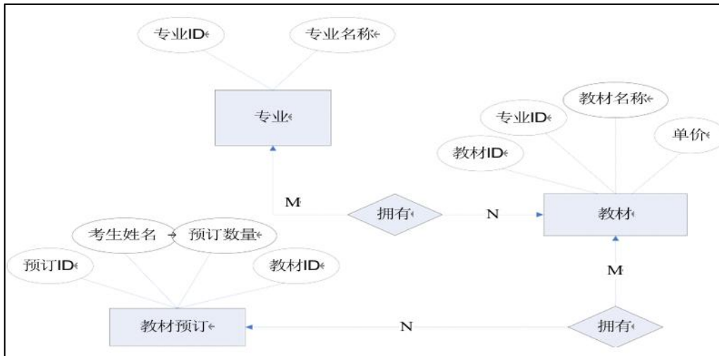
图 2.9.1 E-R 图
