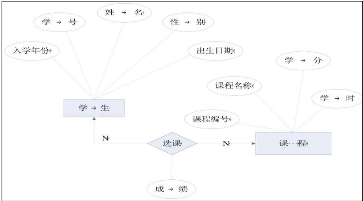
图 2.4.1 E-R 图
