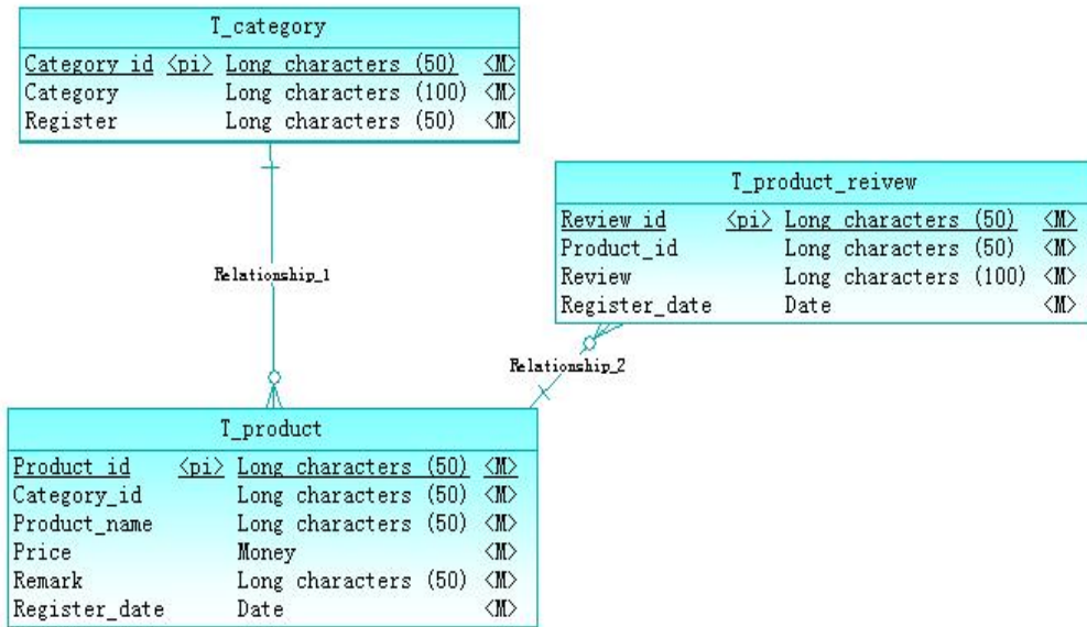
图 2.2.1E-R 图
